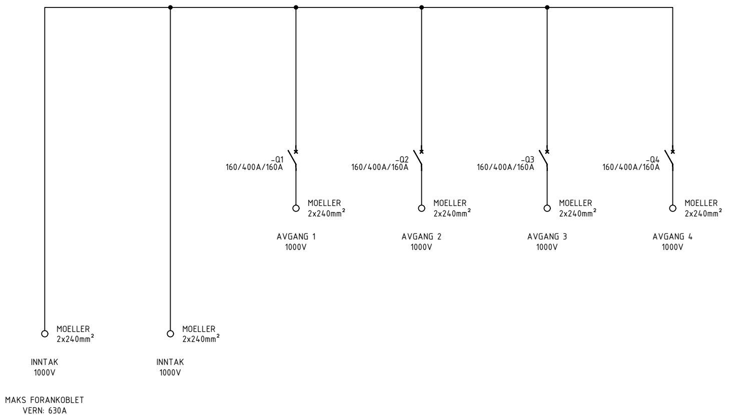
Enlinjeskjema
