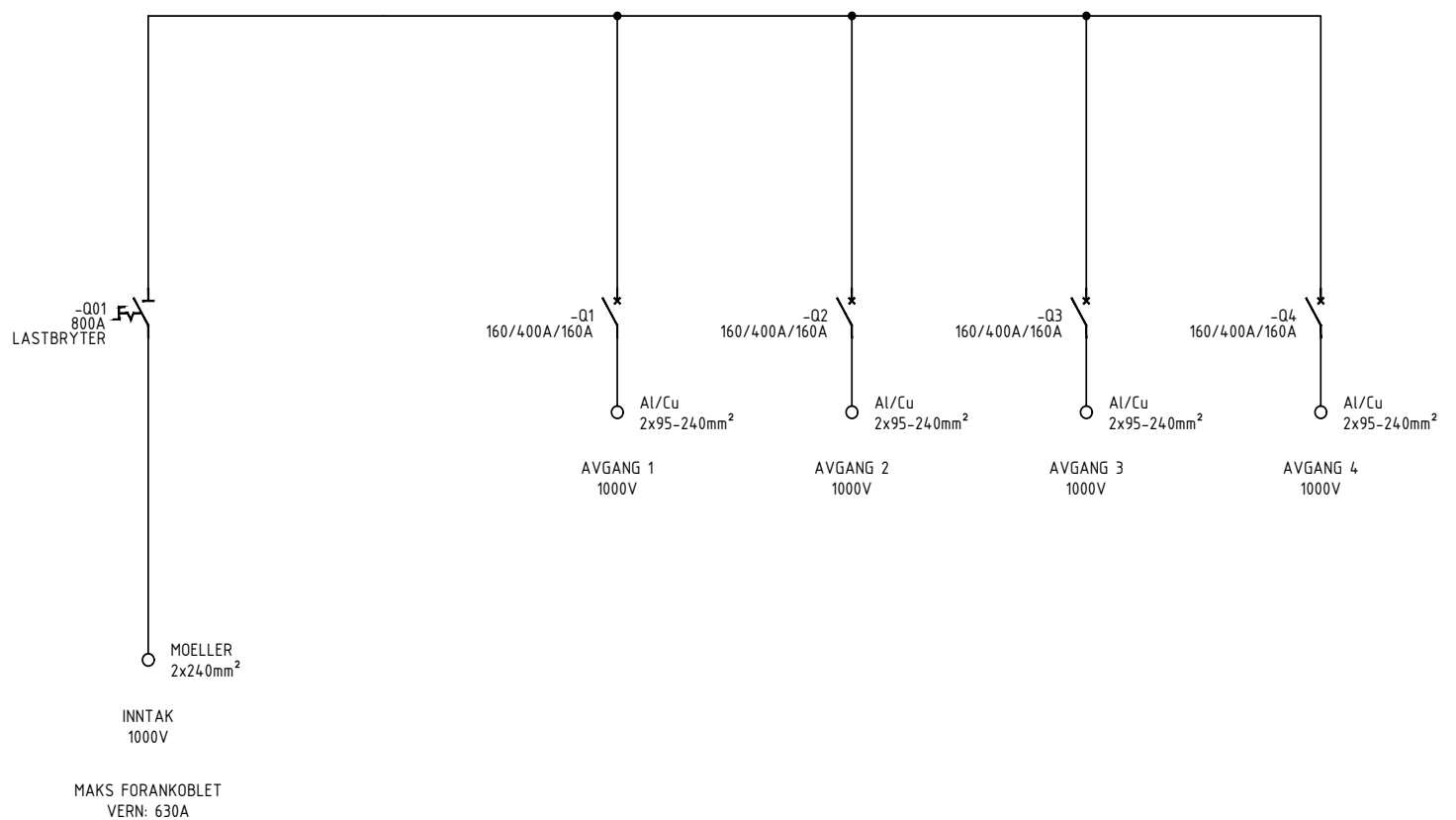
Enlinjeskjema
