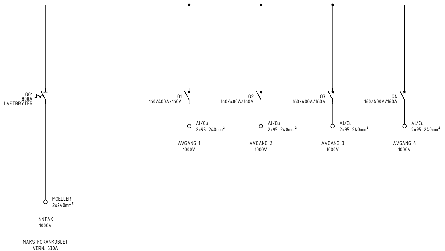
Enlinjeskjema
