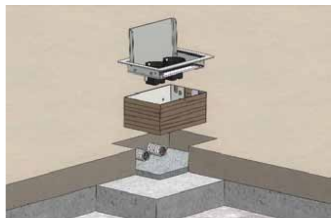
Fjern ramme inkludert koblingsbrett. Tørk boksen og plasser i mørtel.
