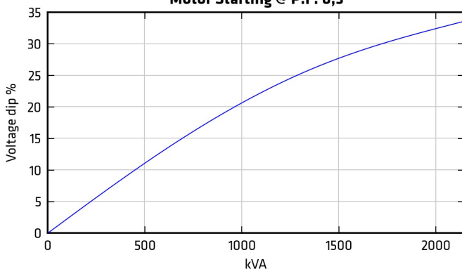
Motor Starting @ P.F. 0,3
