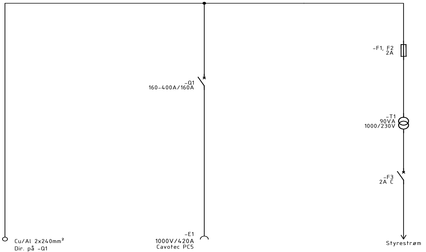
Enlinjeskjema
