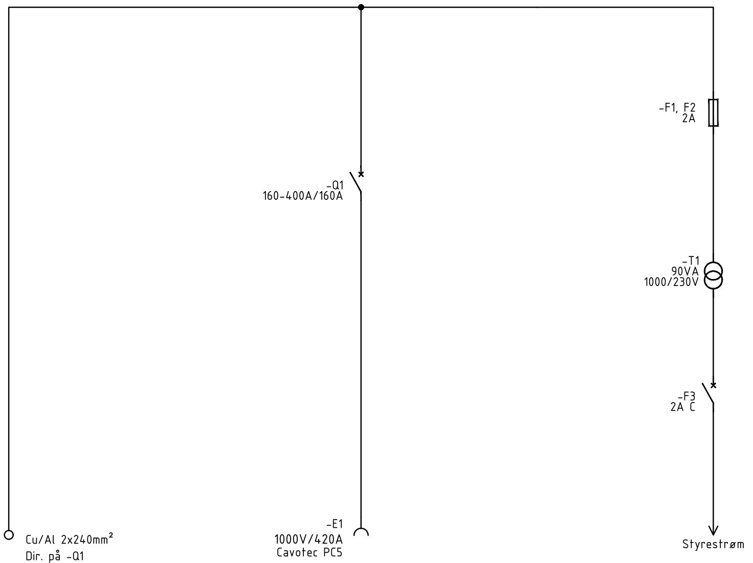
Enlinjeskjema Cavotec
