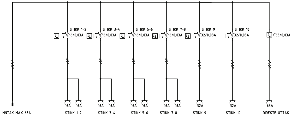
73009 USM-2 63A 01208-R 230V -jordfeilbryter på hver kurs
