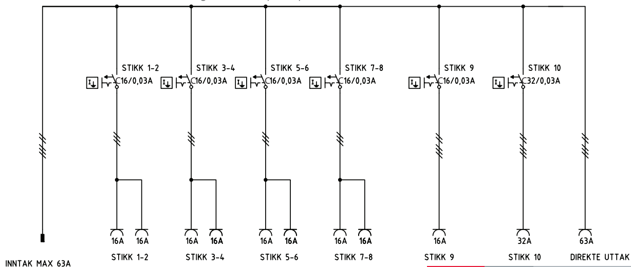
73062 USM-2 63A 01118-R 400V m-jordfeilbryter på hver kurs
